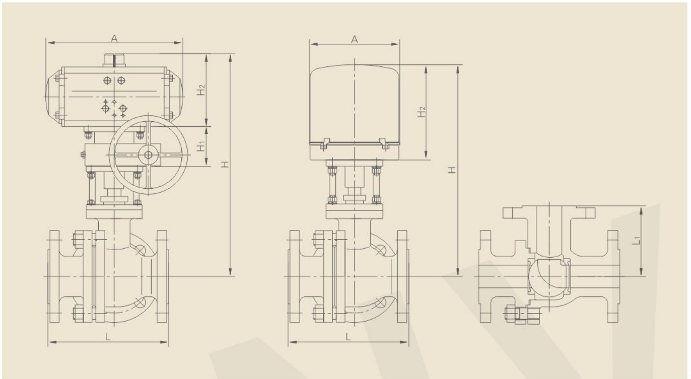
三通球阀外形连接尺寸
